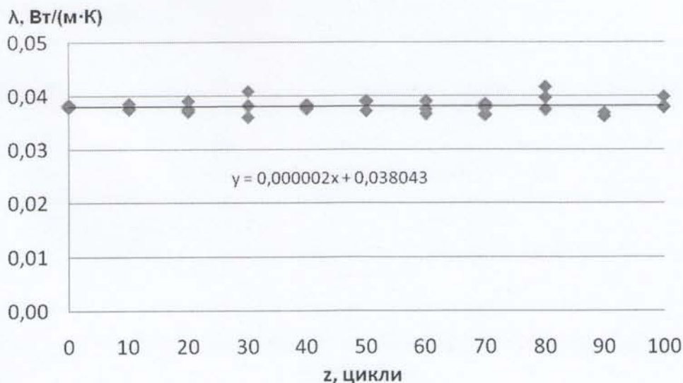
Рисунок 3 – Залежність теплопровідності виробів мінеральної вати ТЕХНО марки ТЕХНОЛАЙТ ЕКСТРА від циклічних впливів
